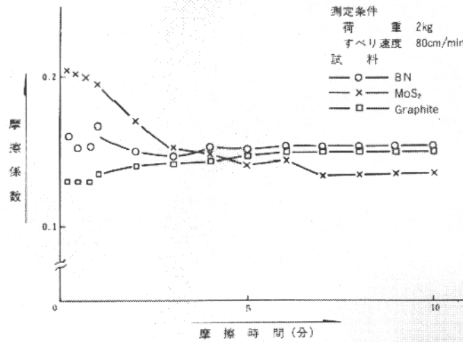
(往復動潤滑試験結果)
