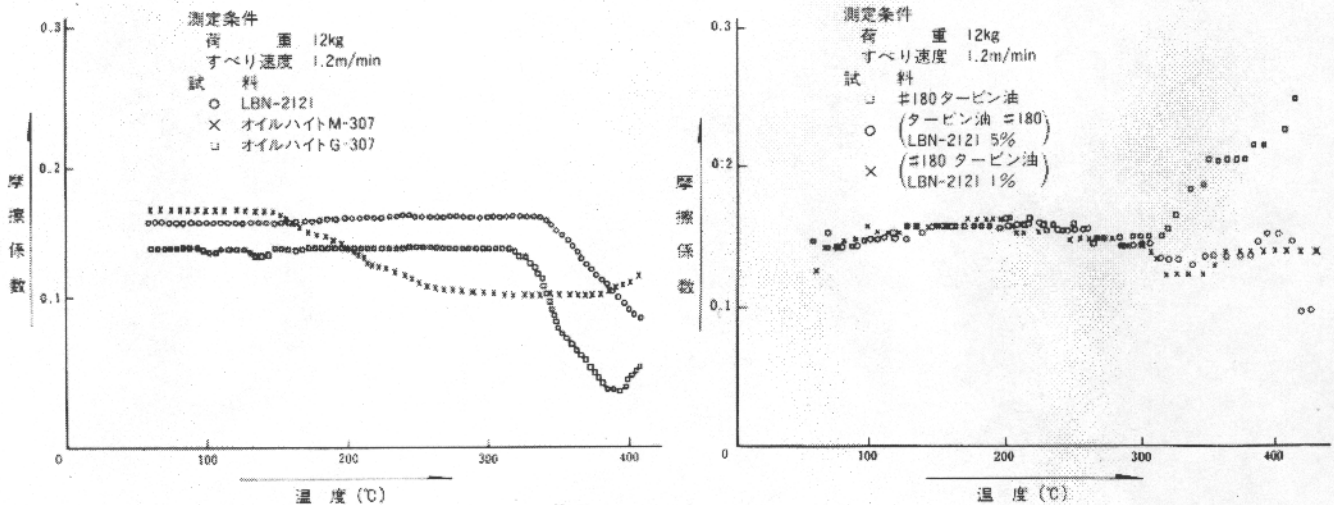
(往復動潤滑試験結果)
